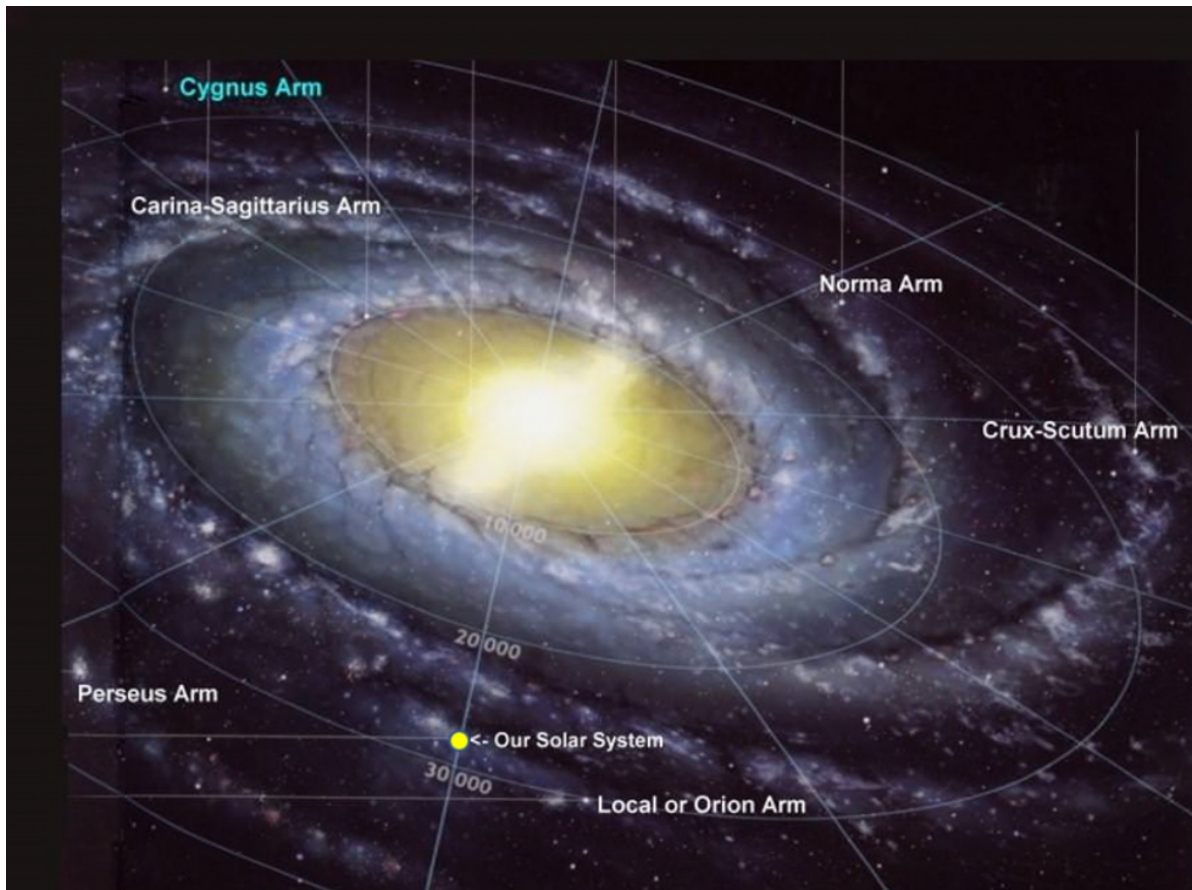
Die Position unseres Sonnensystems in unserer Galaxis, der Milchstrasse
