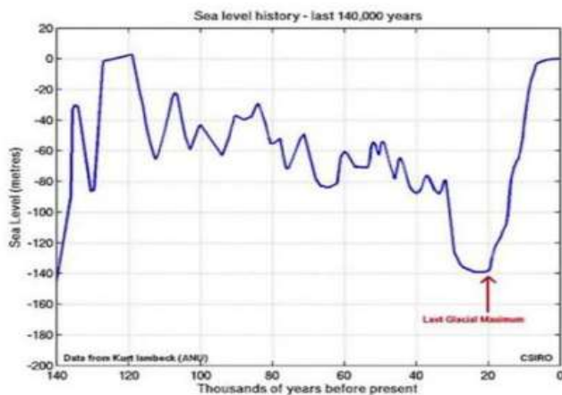
Schwankung des Meeresspiegels in den letzten 140.000 Jahren um ca. 140 m !!
