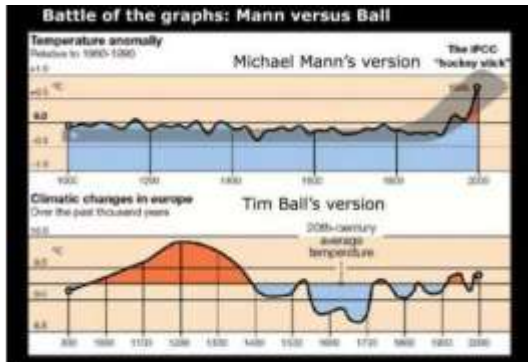
Oben: Manns „Hockeystick“, unten Ball's Klimakurve. Quelle: [unreadable]
