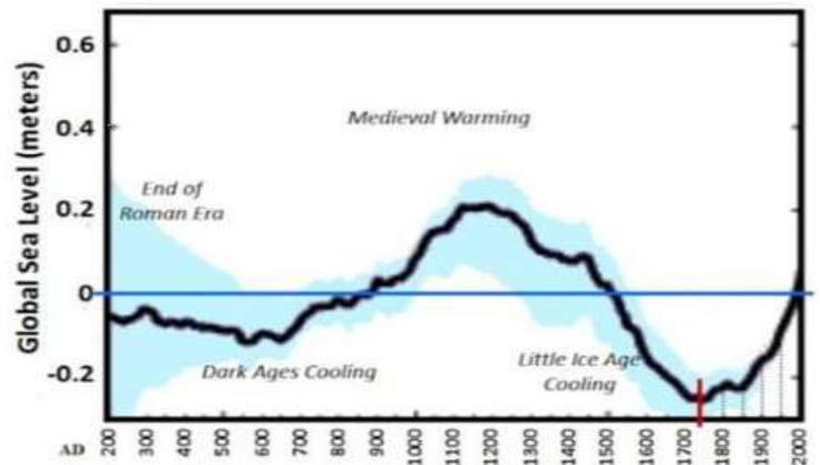
Meeresspiegel vor 800 Jahren ca. 20 cm höher
